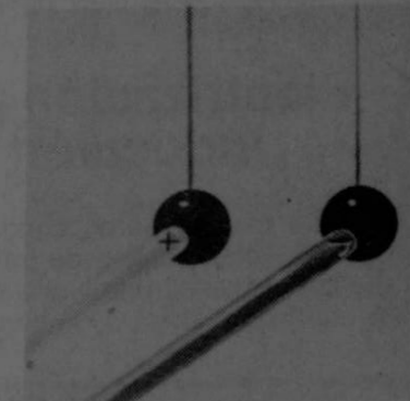
El péndulo tocado con una varilla con carga positiva se vuelve positivo; el tocado con una varilla negativa se torna negativo.
